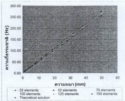
รูปที่ 4 ความสัมพันธ์ระหว่างความถี่ธรรมชาติพื้นฐานและความหนาของเหล็กแผ่นบาง
