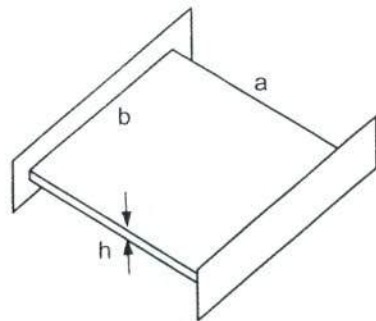
รูปที่ 2 รูปร่างแบบจำลองที่ใช้ในการวิเคราะห์
