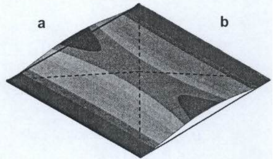
รูปที่ 3 รูปร่างโหมด (Mode Shape) ลำดับที่ 1 ที่เกิดขึ้นในการสั่นสะเทือนของแบบจำลอง
