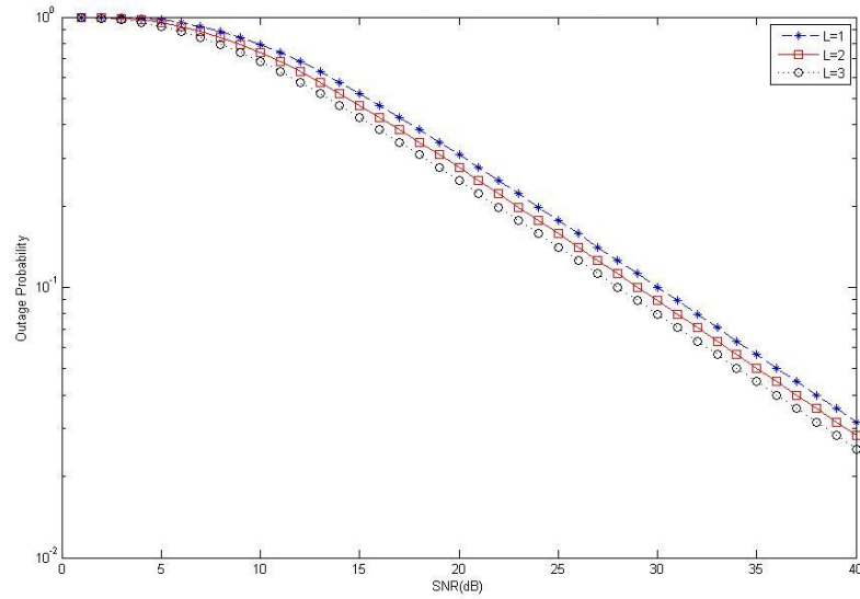
รูปที่ 4.16 Outage Probability ของ Nakagami กรณีที่เพิ่มจุดรับสัญญาณ
